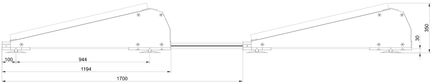
Enkele opstelling met rijafstand van 1890 mm
